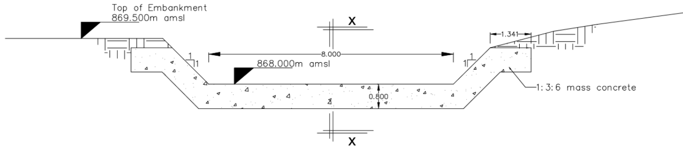
SPILLWAY CONCRETE SILL (Scale: 1:40)
